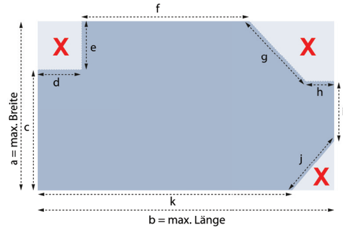
Beispiel-Zeichnung: Form mit drei geraden Anpassungen X
